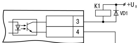
Рисунок 16 – Схема подключения нагрузки к ВУ типа К
