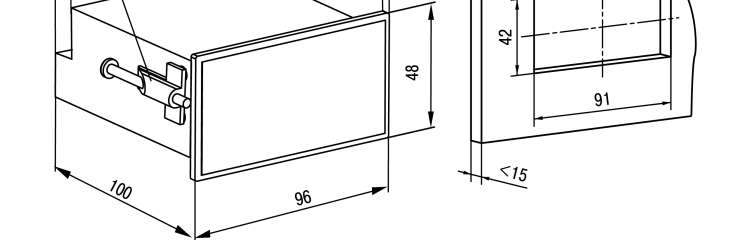
Рисунок 7 – Габаритные размеры корпуса Щ2
