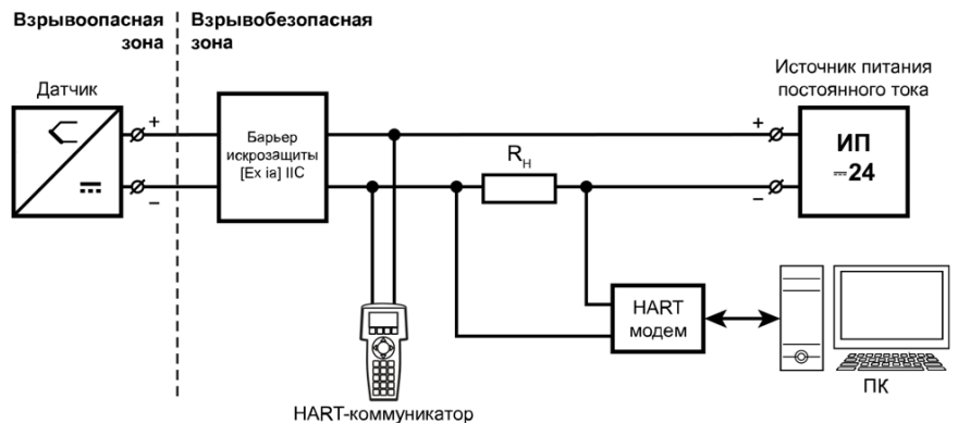
Рисунок 7 – Пример системы с HART-коммуникатором
