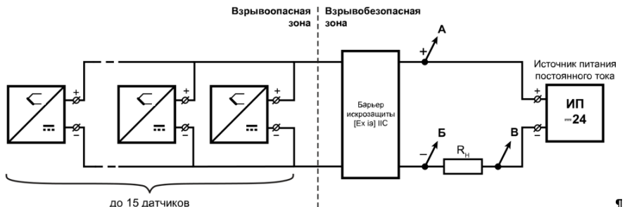
Рисунок 8 – Пример системы с параллельным подключением датчиков
