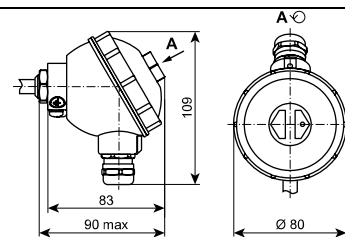
Рисунок 1 – Габаритный чертёж коммутационной головки
