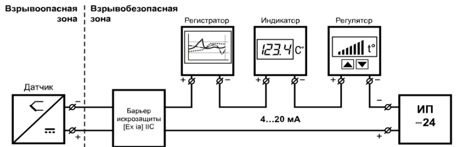
Рисунок 6 – Пример системы
