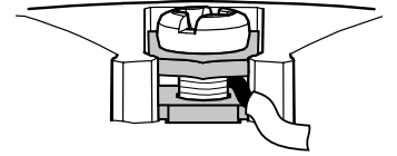
Рисунок 5 – Монтаж провода
