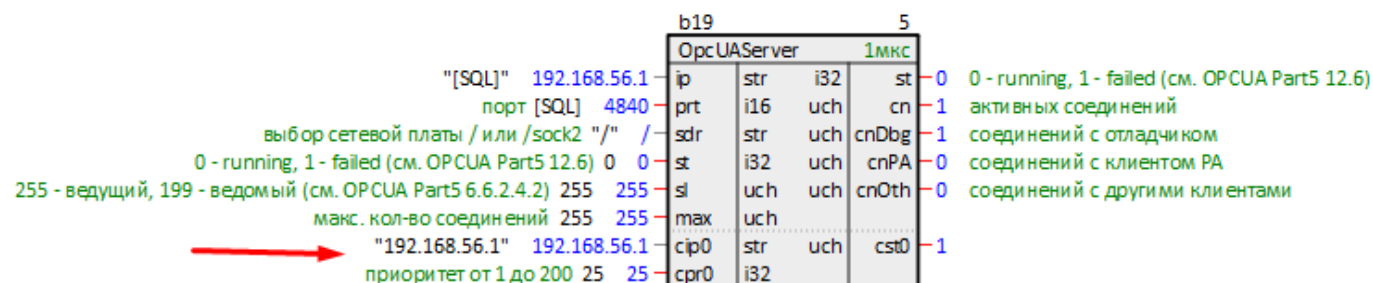
Рисунок 3.17 – OpcUAServer с разрешенным IP-адресом
