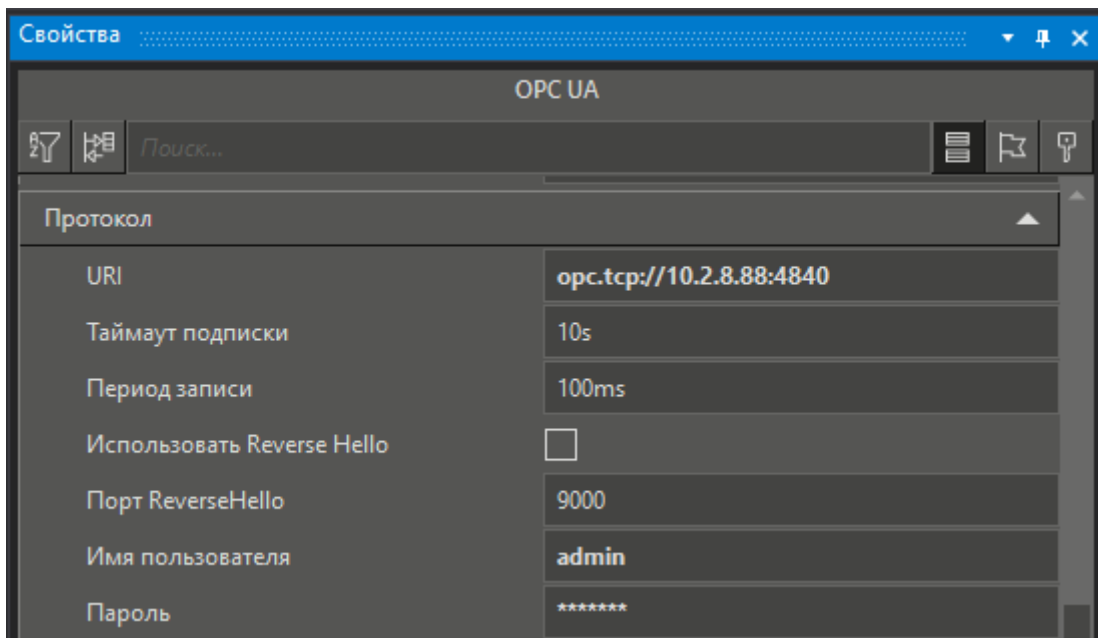
Рисунок 6.7 – Свойства OPC UA
