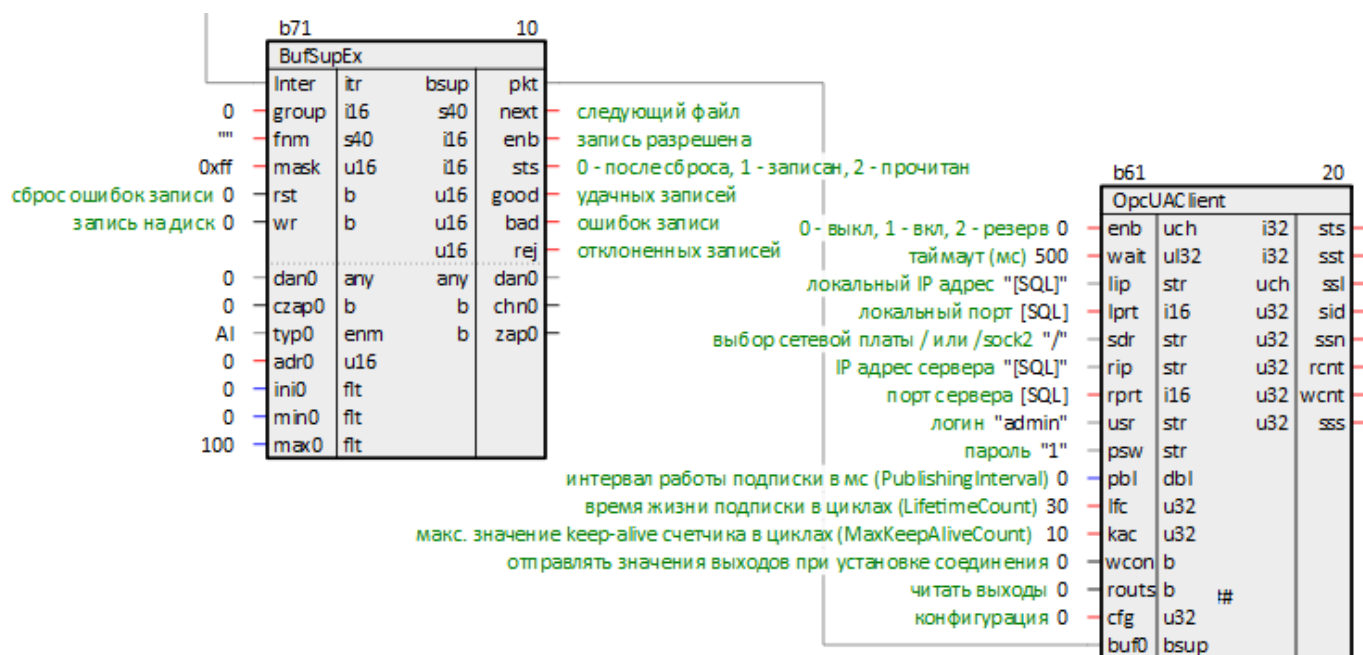
Рисунок 5.3 – Подключение BufSupEx к OpcUAClient
