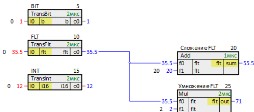
Рисунок 6.10 – Изменение данных в программе ПЛК
