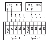
Рисунок 4 – Схема подключения дискретных датчиков с питанием 24 В к входам типа «Д»
