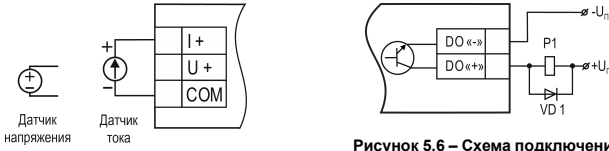
Рисунок 5.5 – Схемы подключения входных сигналов
