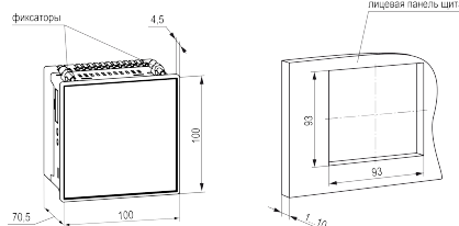
Рисунок 2 – Габаритные размеры и монтажного отверстия в щите
