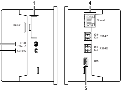
Рисунок 19 – Описание боковых поверхностей
