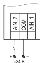
Рисунок 4 – Подключение дискретных датчиков к универсальным входам типа "TRM"
