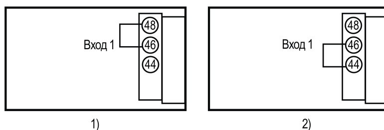
Рисунок 7.7 – Установка переключателя
