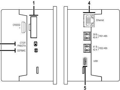
Рисунок 20 – Описание боковых поверхностей
