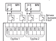
Рисунок 3 – Схема подключения к дискретным входам трехпроводных дискретных датчиков, имеющих выходной транзистор р-р-р-типа с открытым коллектором для сигналов 24 В
