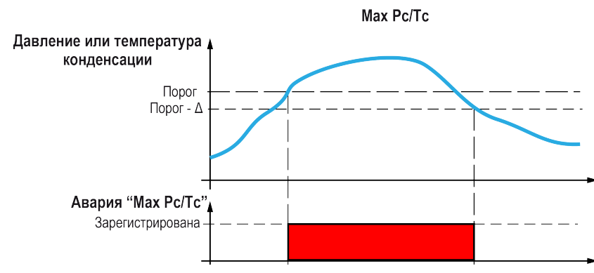
Рисунок 8.16 – Поясняющая диаграмма регистрации прибором аварии по превышению максимального порога давления или температуры конденсации
