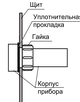
Рисунок 2 – Монтаж прибора
