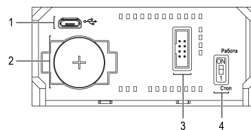
Рисунок 12 – Лицевая панель под крышкой
