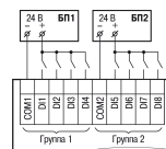
Рисунок 4 – Схема подключения дискретных датчиков с питанием 24 В к входам типа «Д»
