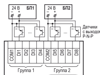
Рисунок 3 – Схема подключения к дискретным входам трехпроводных дискретных датчиков, имеющих выходной транзистор р-п-р-типа с открытым коллектором для сигналов 24 В
