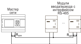
Рисунок 14 – Типовая схема подключения в режиме Master
