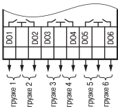
Рисунок 10 – Схема подключения ВЭ типа «Р»
