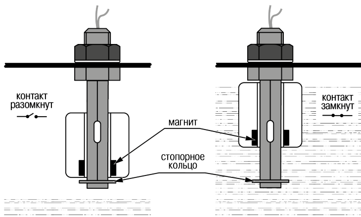
Рисунок 5.1 – Принцип действия
