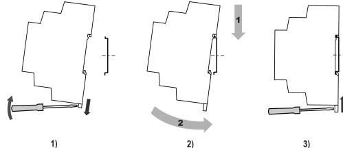
Рисунок 1 – Установка прибора
