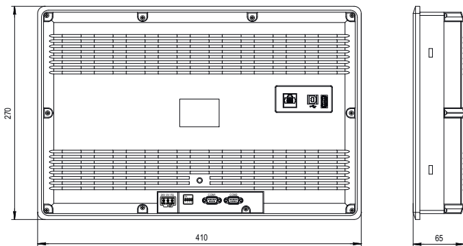
Рисунок 2 – Габаритные размеры СП315
