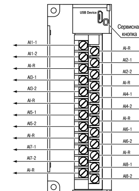
Рисунок 1 – Назначение контактов клемника
