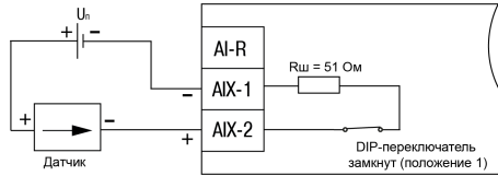
Рисунок 6 – Схема подключения датчиков с унифицированным выходным сигналом тока 0...20 мА и 0...5 мА по двухпроводной схеме
