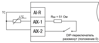
Рисунок 3 – Схема подключения ТС по трехпроводной схеме
