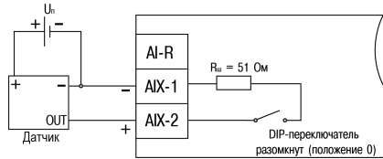
Рисунок 5 – Схема подключения датчиков с унифицированным выходным сигналом напряжения -50...+50 мВ и -1...+1 В по трехпроводной схеме
