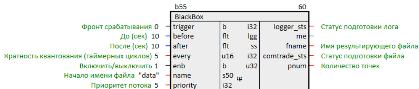
Рисунок 4.2 – Черный ящик (BlackBox)
