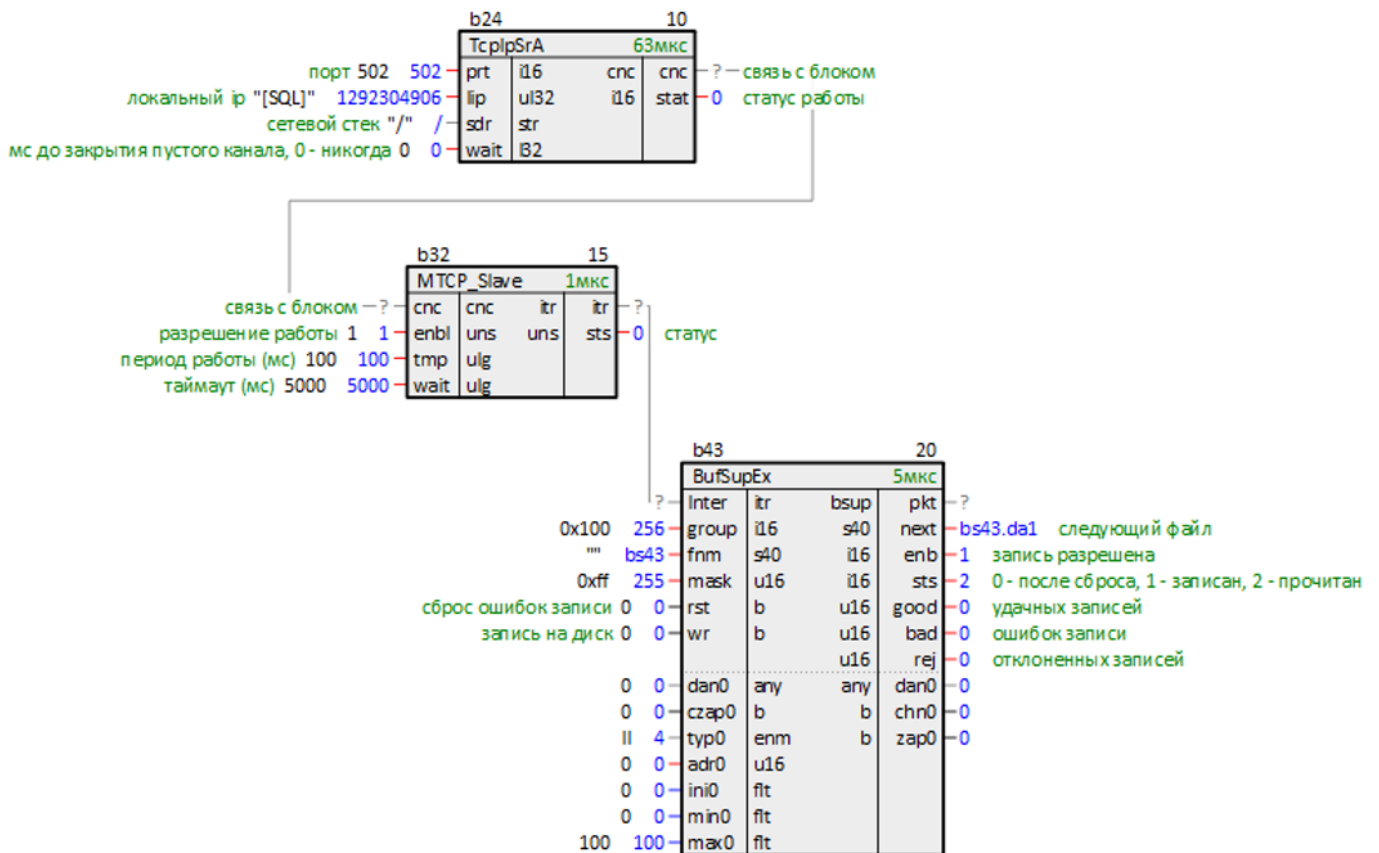
Рисунок 5.14 – Подключение BufSupFltEx к Modbus TCP Slave
