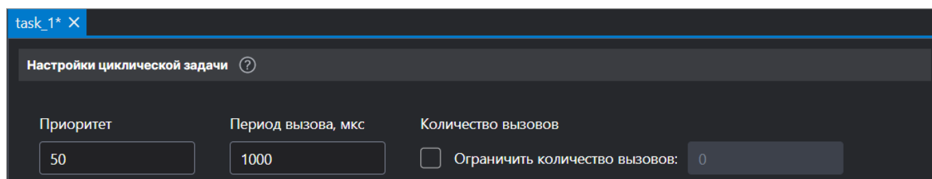
Рисунок 4.32 – Настройки циклической задачи
