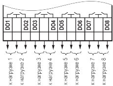
Рисунок 9 – Схема подключения к выходам типа «Р»
