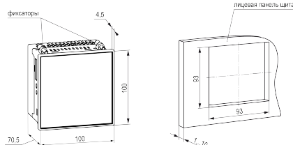
Рисунок 2 – Габаритные размеры и монтажного отверстия в щите
