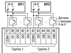
Рисунок 5 – Подключение датчиков с выходным транзистором р-п-р-типа
