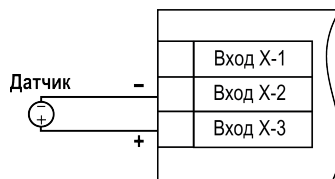
Рисунок 5.19 – Схема подключения активного датчика с выходом в виде напряжения -50\dots+50 мВ или 0\dots1 В
