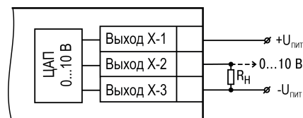
Рисунок 5.29 – Схема подключения нагрузки к ВУ типа «У»
