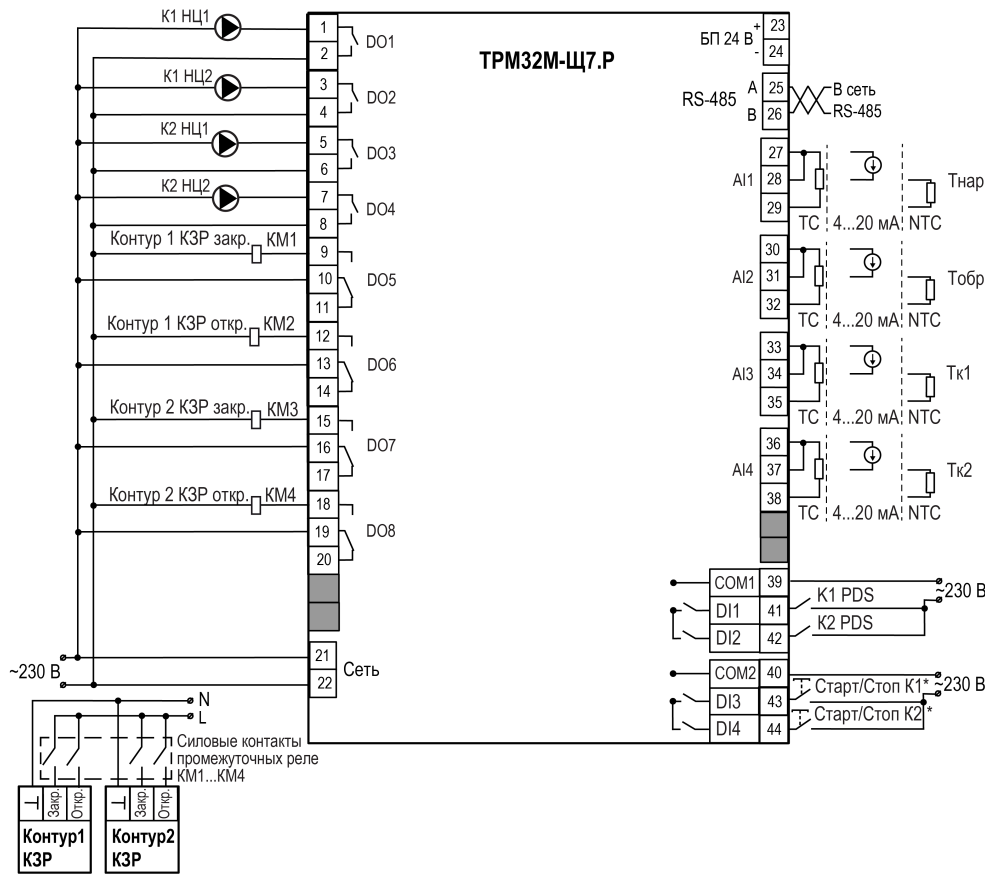
Рисунок 7.12 – Схема подключения ТРМ32М-Щ7.Р
