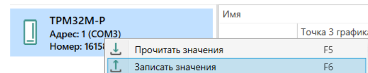
Рисунок 6.19 – Контекстное меню
