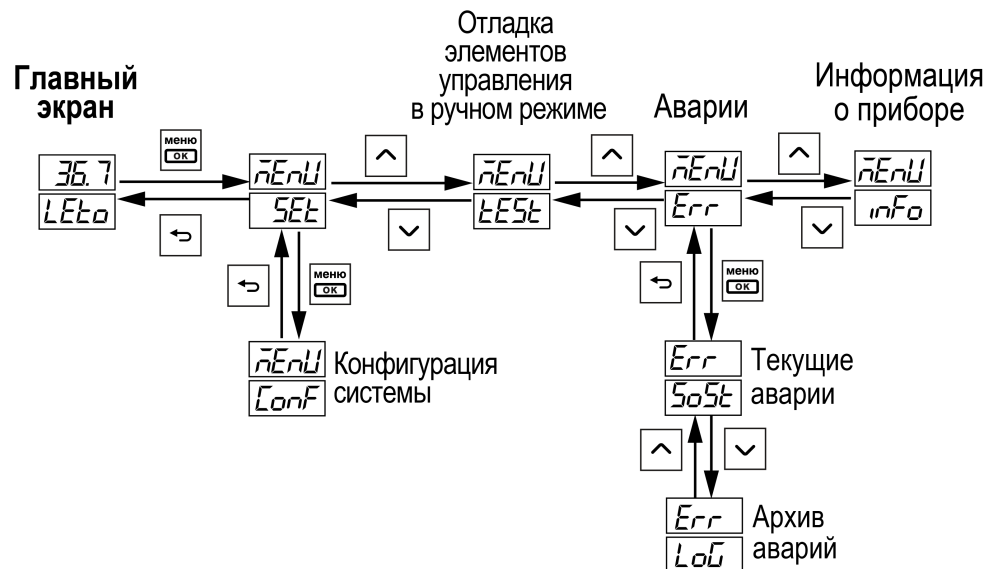
Рисунок 8.3 – Структура меню
