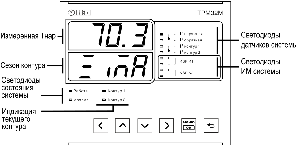
Рисунок 8.11 – Главный экран
