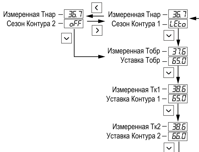
Рисунок 8.2 – Главный экран
