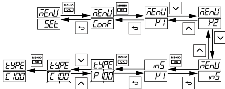
Рисунок 10.1 – Настройка параметра с помощью кнопок
