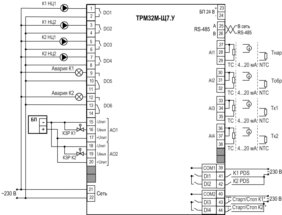
Рисунок 7.14 – Схема подключения ТРМ32М-Ц7.У
