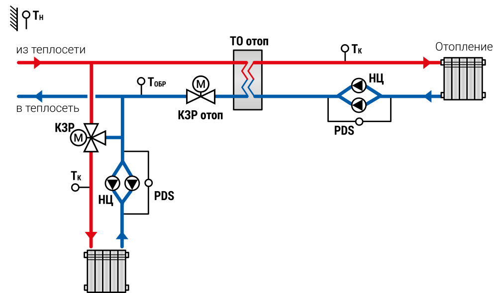
Рисунок 5.3 – Схема независимого контура отопления и зависимого смесительного контура отопления
