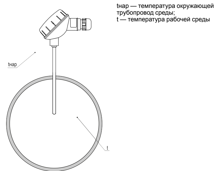
Рисунок А.6 – Пример неверного монтажа датчика
