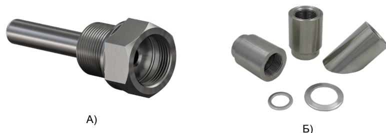
Рисунок А.7 – Арматура для датчиков: А) защитная гильза, Б) приварные бобышки
