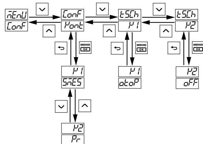
Рисунок 8.4 – Конфигурация системы
