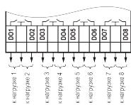
Рисунок 8 – Схема подключения к выходам типа «P»
