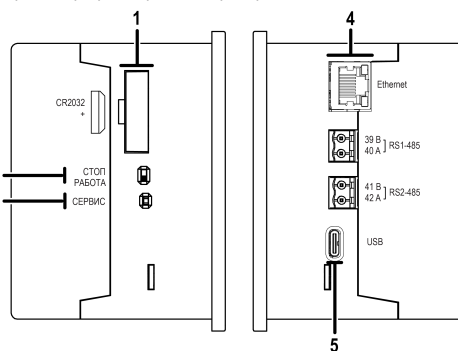
Рисунок 15 – Описание боковых поверхностей
