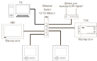
Рисунок 10 – Подключение по схеме «Звезда»
