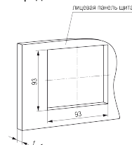
Рисунок 2 – Габаритные размеры и монтажного отверстия в щите
