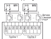
Рисунок 3 – Схема подключения к дискретным входам трехпроводных дискретных датчиков, имеющих выходной транзистор р-п-р-типа с открытым коллектором для сигналов 24 В
