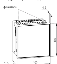
Рисунок 2 – Габаритные размеры и монтажного отверстия в щите
