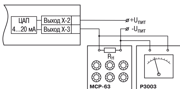
Рисунок 8.8 – Подключение ВУ1 типа И ( R_H=500 \text{ Ом} )
