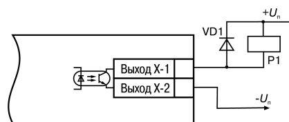
Рисунок 5.12 – Схема подключения нагрузки к ВУ1 типа К
