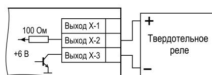
Рисунок 5.13 – Схема подключения нагрузки к ВУ типа Т
