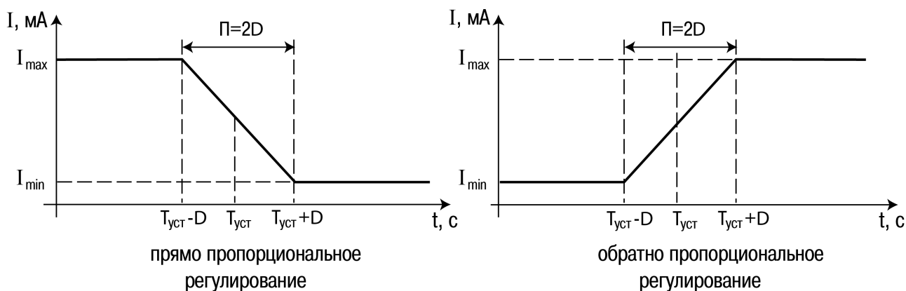
Рисунок 7.8 – Виды регулирования
