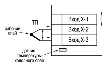
Рисунок 5.7 – Схема подключения термопары
