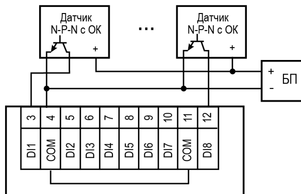
Рисунок 3 – Схема подключения трехпроводных дискретных датчиков, имеющих выходной транзистор п-р-п типа с открытым коллектором
