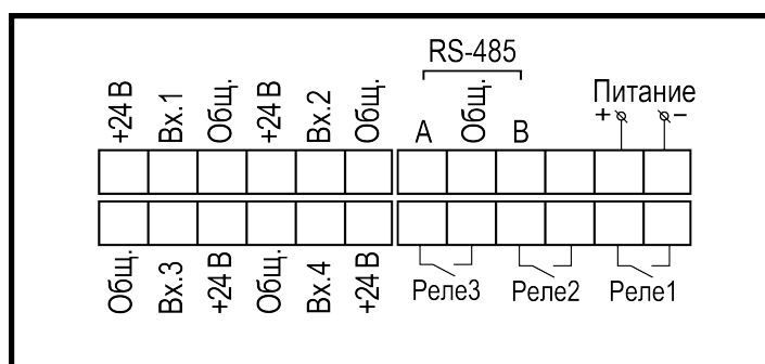
Рисунок 6.2 – Клеммник САУ-У2.Х.Щ12
