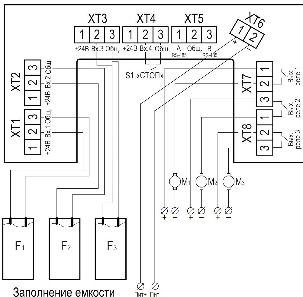
Рисунок 9.4 – Схема подключения для алгоритма 06
