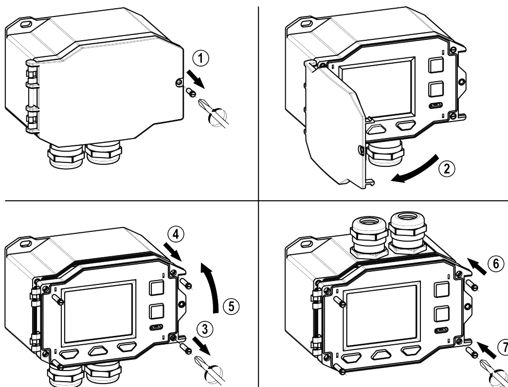
Рисунок 5.5 – Поворот корпуса CAU-U2.X.H4
