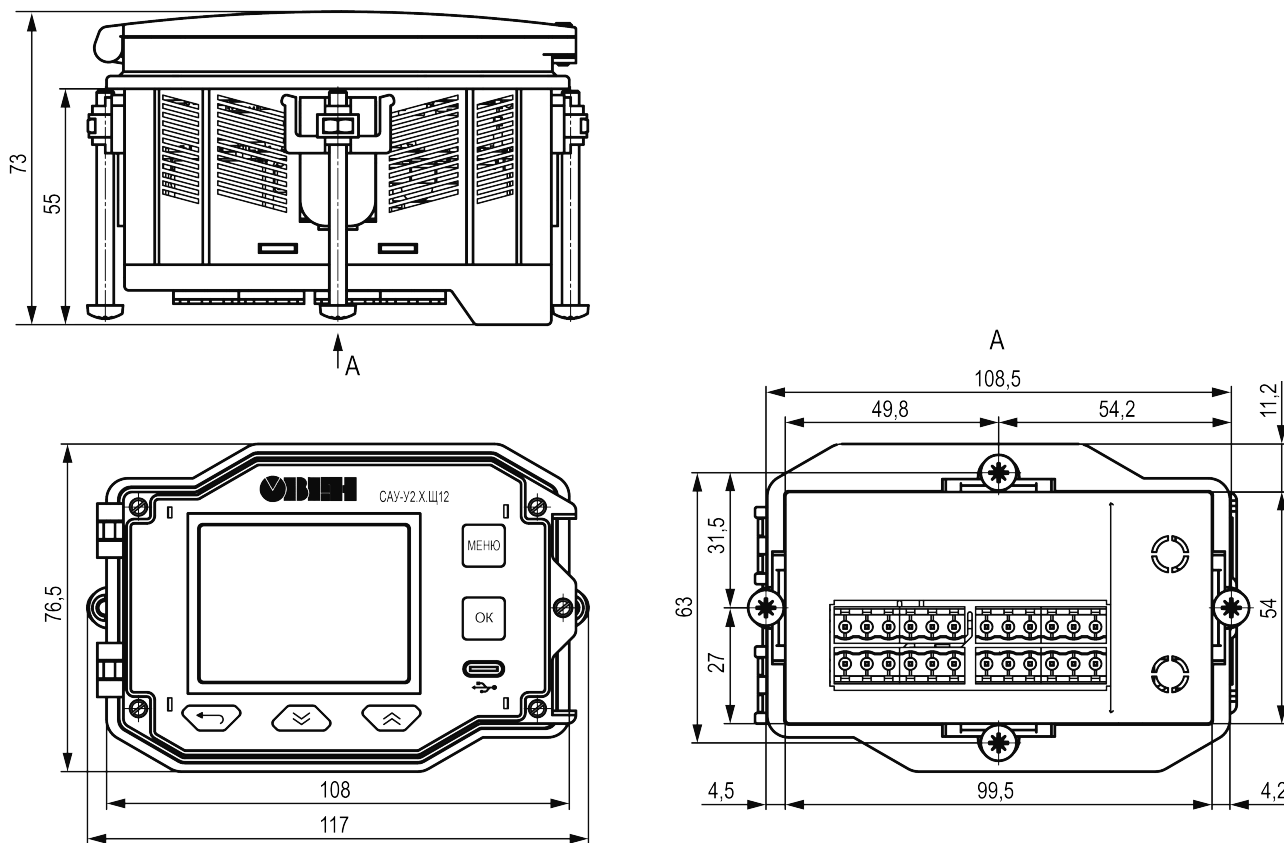
Рисунок 5.2 – Габаритные и присоединительные размеры CAU-Y2.X.Щ12
