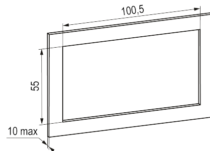
Рисунок 5.6 – Размеры выреза под монтаж САУ-У2.Х.Щ12
