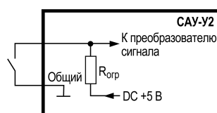
Рисунок 6.6 – Схема подключения механических контактных датчиков
