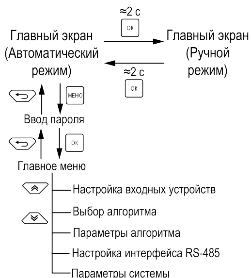
Рисунок 8.1 – Структура меню САУ-У2.Х.Н4/САУ-У2.Х.Щ12
