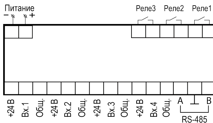
Рисунок 6.3 – Клеммник САУ-У2.Х.Д7
