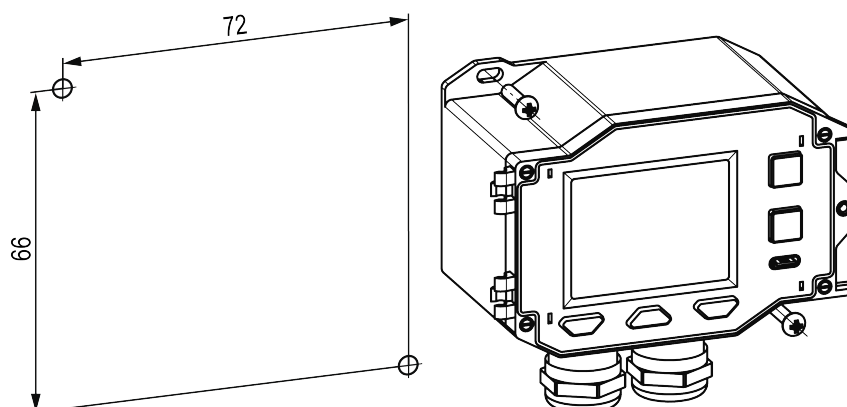
Рисунок 5.4 – Монтаж CAU-U2.X.H4
