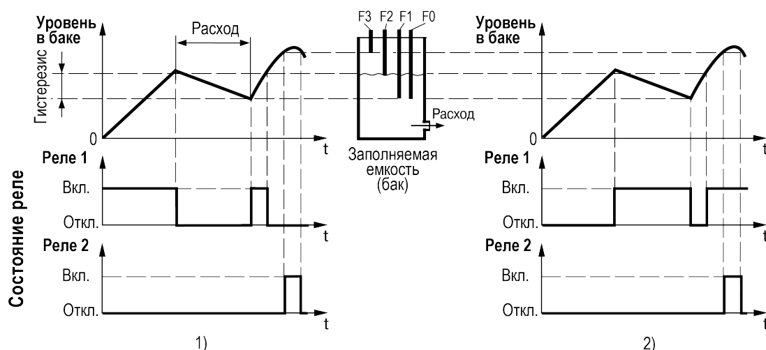
Рисунок 9.2 – Графики работы прибора: 1) заполнение, 2) осушение
