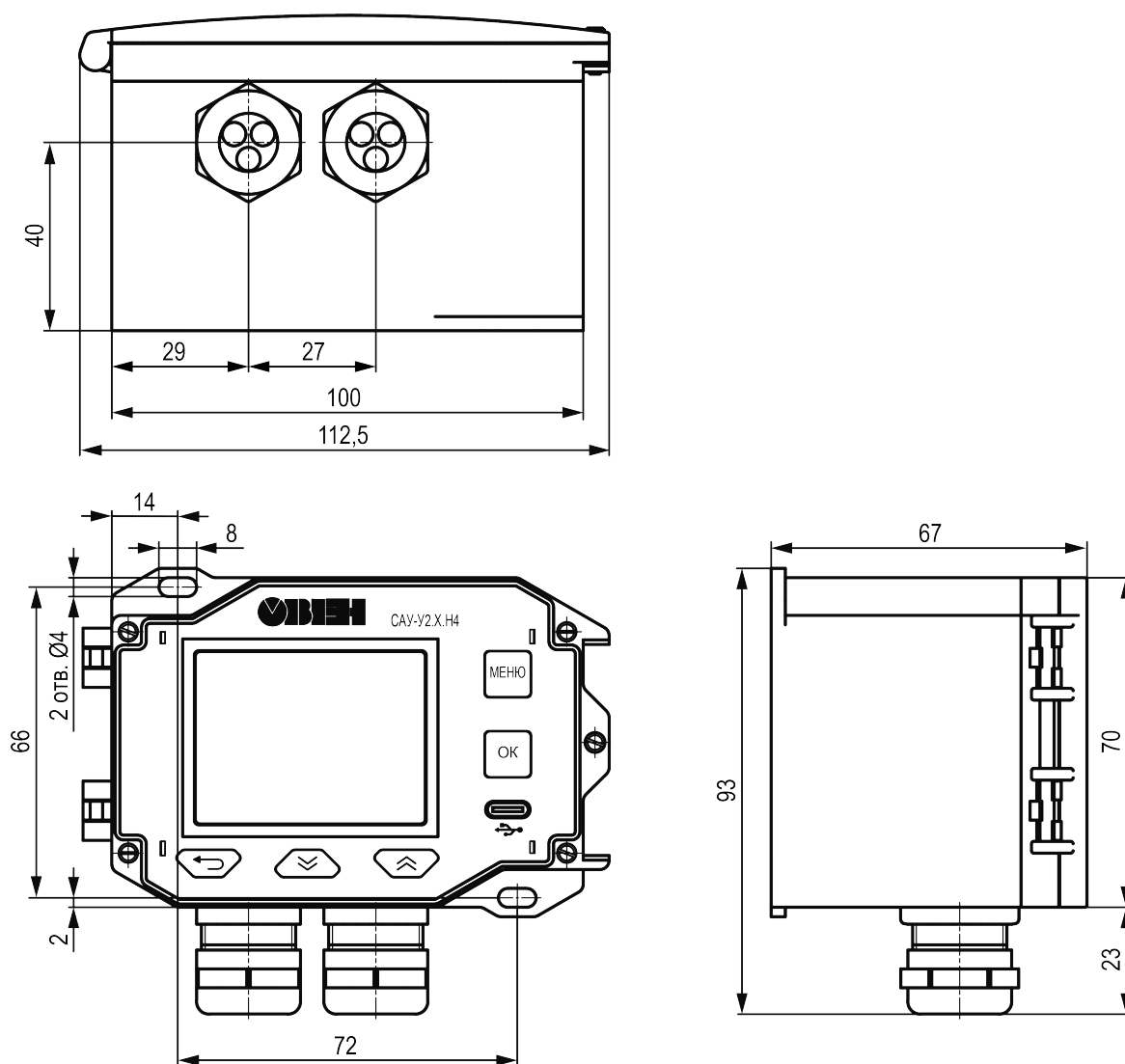
Рисунок 5.1 – Габаритные и присоединительные размеры САУ-У2.Х.Н4
