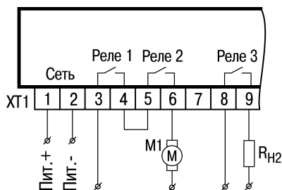
Рисунок 9.16 – Подключение контактов реле 2 в САУ-У2.Х.Н4 для выполнения алгоритма 20 с защитным отключением насоса M1
