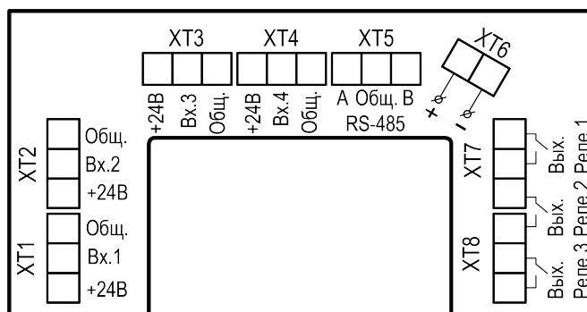
Рисунок 6.1 – Клеммник САУ-У2.Х.Н4
