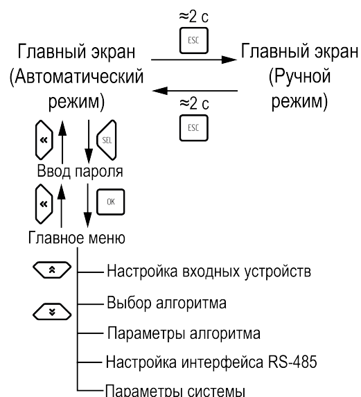
Рисунок 8.2 – Структура меню САУ-У2.Х.Д7
