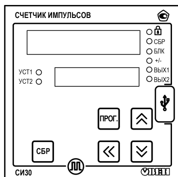
Рисунок 6.2 – Лицевая панель прибора для корпусов настенного Н и щитового Щ1 креплений
