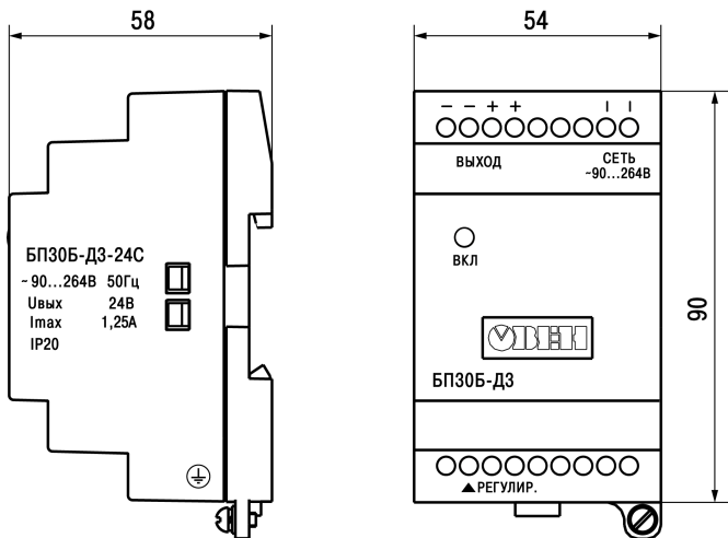
Рисунок 1 - Габаритные размеры прибора
