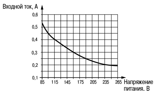
Рисунок 6 - График зависимости входного тока от напряжения питания
