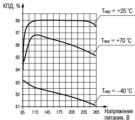
Рисунок 7 - График зависимости КПД от напряжения питания и температуры окружающей среды
