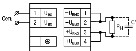
Рисунок 3 - Схема подключения прибора
