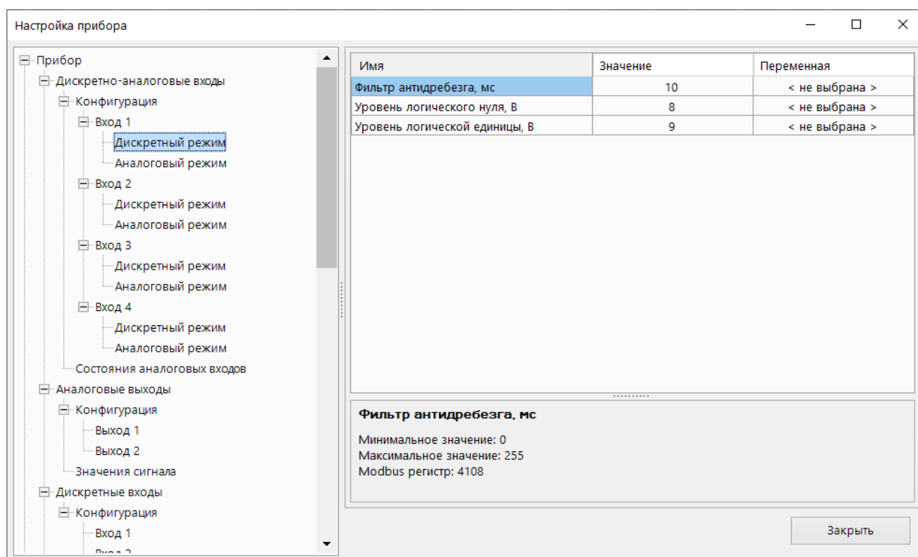
Рисунок 4.6 – Настройки дискретного режима входа типа “ДАТ”
