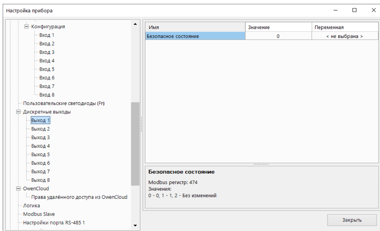
Рисунок 4.15 – Настройка безопасного состояния дискретных выходов
