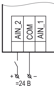
Рисунок 6.8 – Подключение дискретных датчиков
