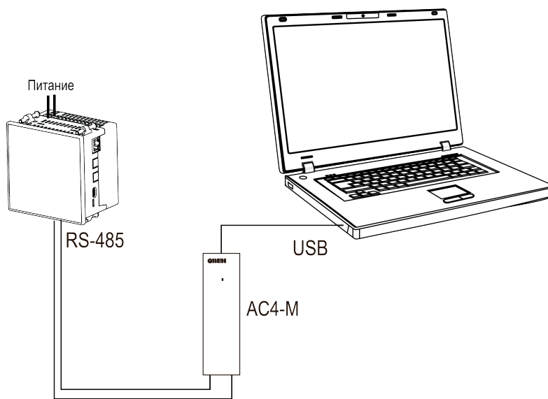
Рисунок 6.30 – Схема подключения прибора к ПК по RS-485
