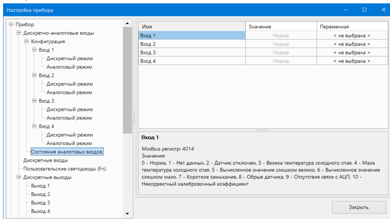
Рисунок 4.9 – Меню кодов ошибок датчиков
