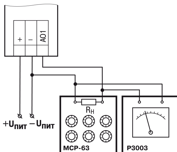
Рисунок В.5 – Схема подключения к ВЭ для юстировки сигналов типа «4...20 мА» ( R_H < 600 \text{ Ом} )
