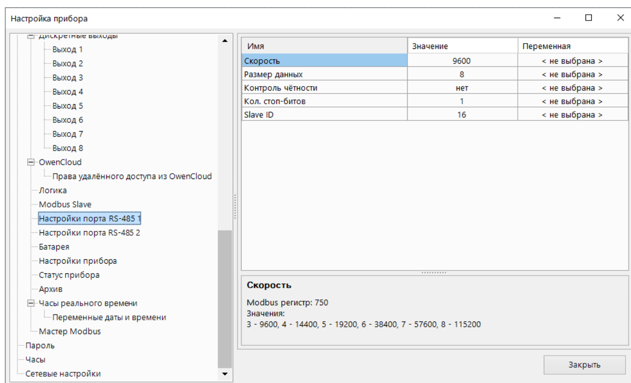
Рисунок 4.22 – Настройки параметров RS-485
