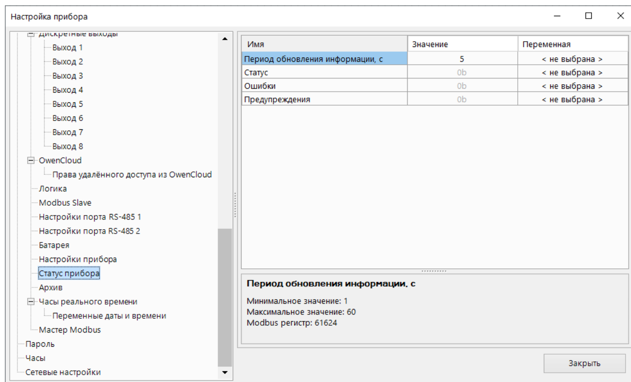
Рисунок 4.38 – Параметры статуса прибора
