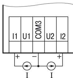
Рисунок 6.17 – Подключение датчиков с выходом в виде тока
