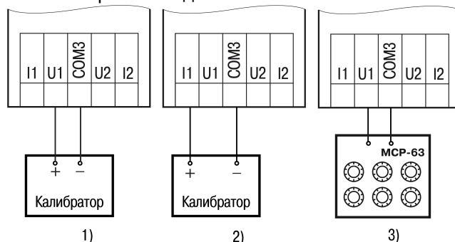
Рисунок В.3 – Подключение источника эталонного сигнала
