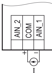
Рисунок 6.6 – Схема подключения датчиков с выходным сигналом силы тока постоянного напряжения от 0 до 20 мА и от 4 до 20 мА
