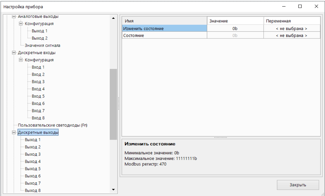
Рисунок 4.14 – Состояние дискретных выходов
