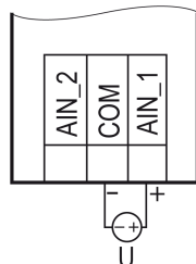
Рисунок 6.4 – Схема подключения датчиков с выходными сигналами постоянного напряжения от -50 до +50 мВ
