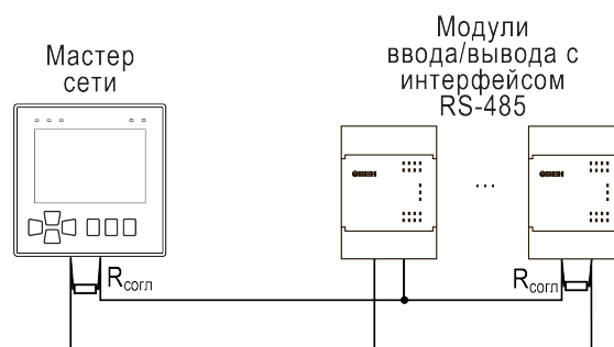
Рисунок 6.25 – Типовая схема подключения в режиме Master
