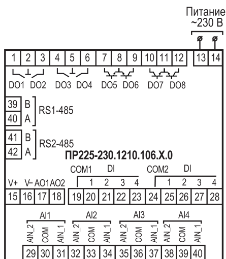
Рисунок А.14 – Расположение контактов для PR225–230.1210.106.X.0
