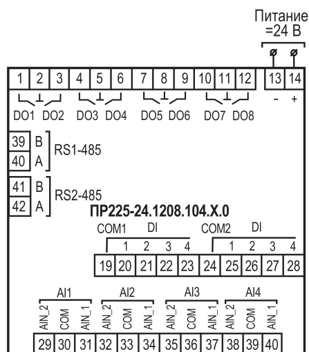
Рисунок А.13 – Расположение контактов для ПР225–24.1208.104.X.0
