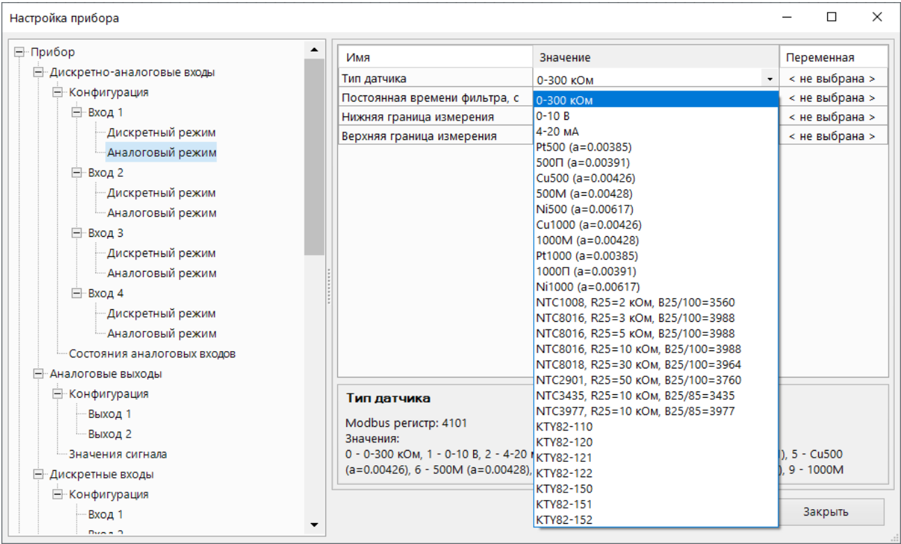
Рисунок 4.5 – Меню настройки аналогового режима входа типа “ДАТ”
