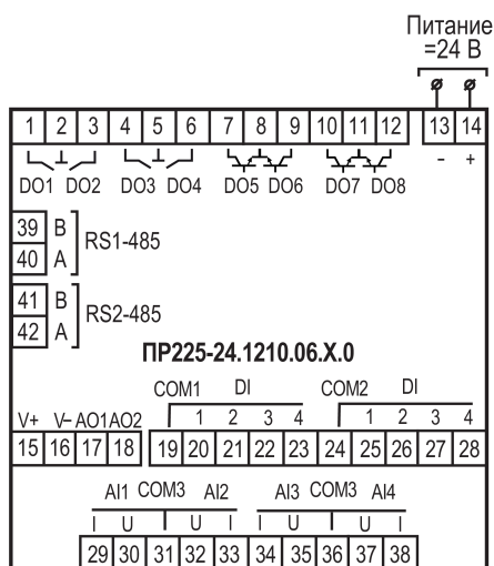
Рисунок А.9 – Расположение контактов для PR225–24.1210.06.X.0
