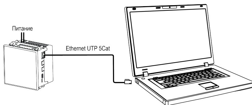
Рисунок 6.29 – Схема подключения прибора к ПК по Ethernet
