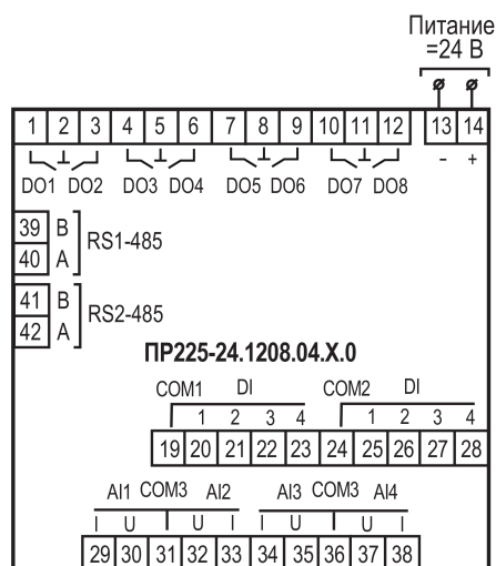
Рисунок А.8 – Расположение контактов для ПР225–24.1208.04.X.0
