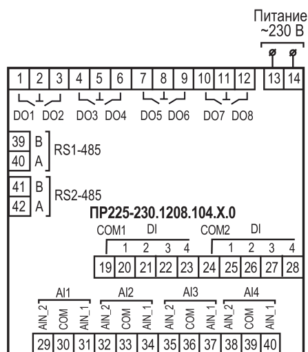
Рисунок А.12 – Расположение контактов для ПР225–230.1208.104.X.0
