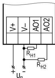
Рисунок 6.22 – Подключение аналогового выхода, находящегося в режиме источника напряжения
