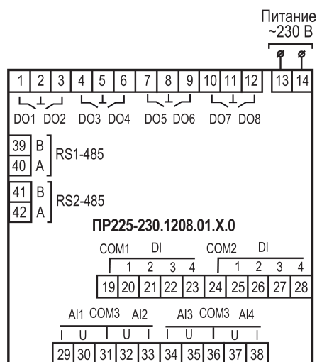
Рисунок А.2 – Расположение контактов для PR225–230.1208.01.X.0
