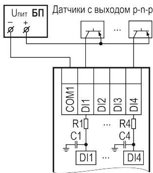
Рисунок 6.13 – Подключение к входам типа «Д» датчиков с выходом р-п-р
