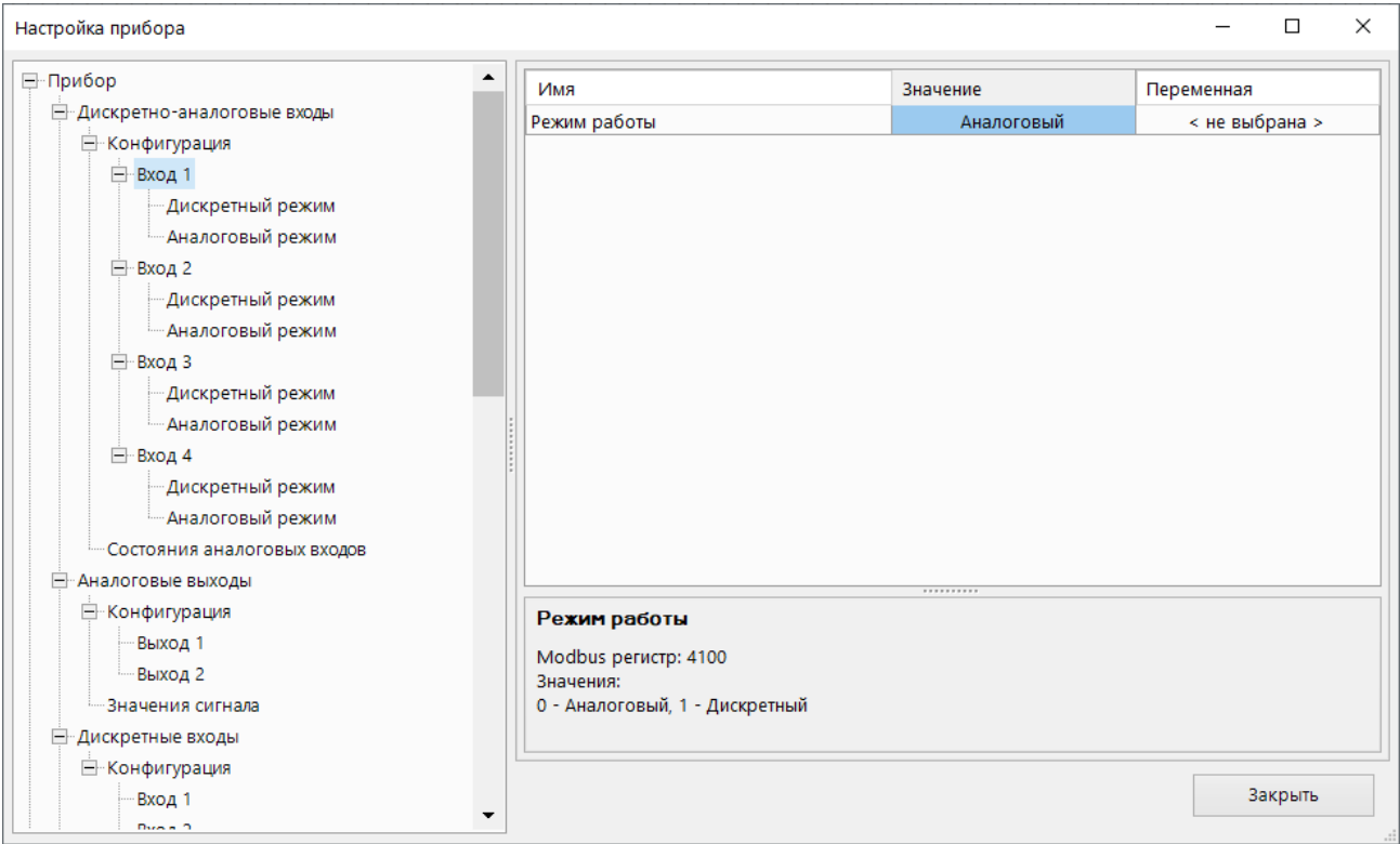
Рисунок 4.4 – Настройка режима работы входа типа “ДАТ”
