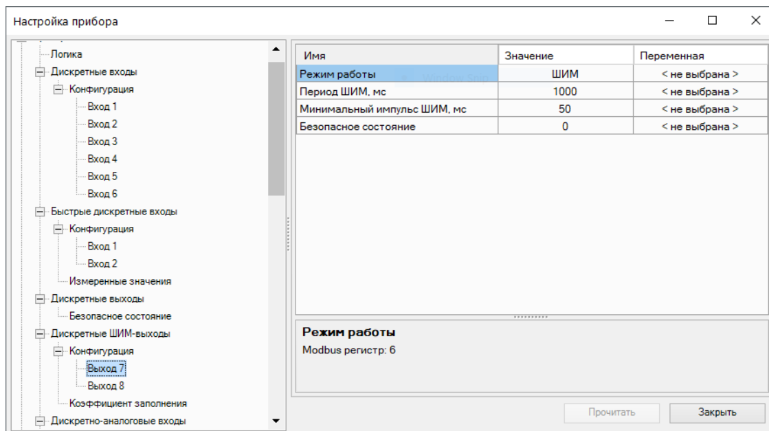
Рисунок 4.17 – Настройка параметров работы выхода типа «КТ» в режиме ШИМ
