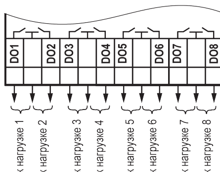
Рисунок 6.20 – Схема подключения ВЭ типа «Р»
