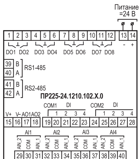
Рисунок А.11 – Расположение контактов для PR225–24.1210.102.X.0
