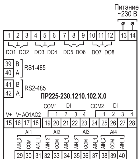
Рисунок А.10 – Расположение контактов для ПР225–230.1210.102.X.0
