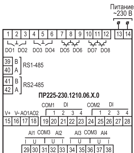
Рисунок А.5 – Расположение контактов для PR225–230.1210.06.X.0
