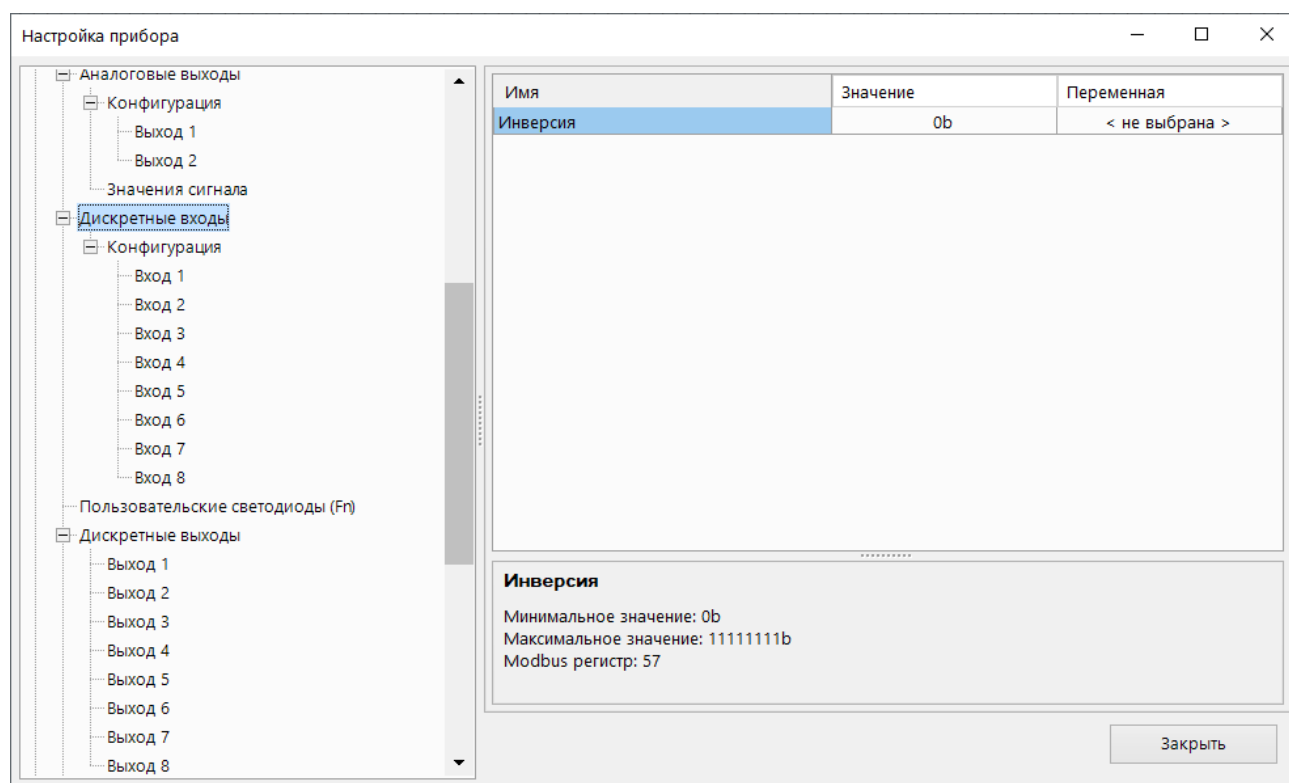
Рисунок 4.10 – Настройка инверсии дискретных входов
