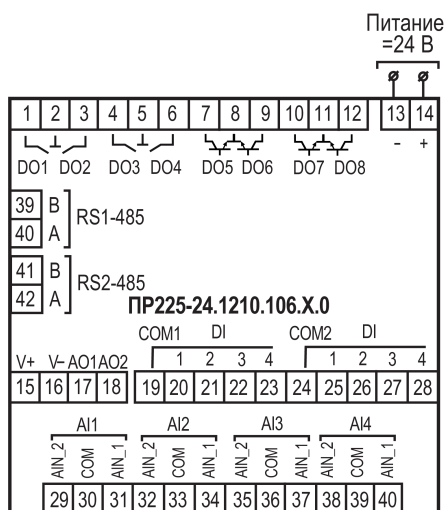
Рисунок А.15 – Расположение контактов для ПР225–24.1210.106.X.0
