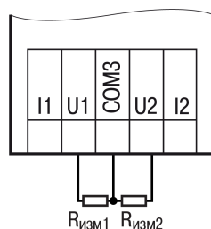
Рисунок 6.19 – Подключение резистивных датчиков
