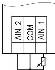
Рисунок 6.7 – Подключение резистивных датчиков
