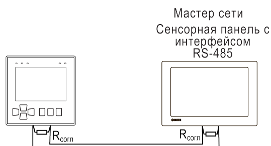
Рисунок 6.24 – Типовая схема подключения в режиме Slave
