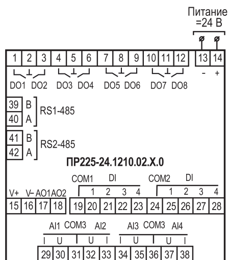
Рисунок А.7 – Расположение контактов для PR225–24.1210.02.X.0
