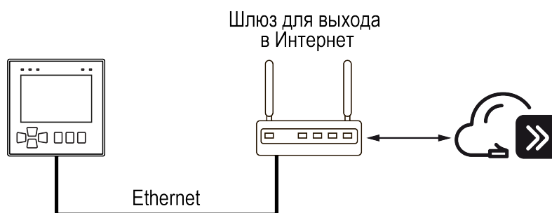
Рисунок 6.27 – Подключение к OwenCloud
