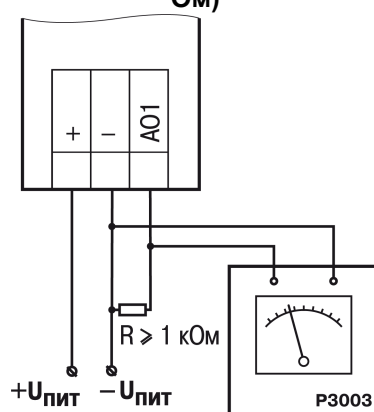
Рисунок В.6 – Схема подключения нагрузки к ВЭ для юстировки сигналов типа «0...10 В» ( R_H > 600 \text{ Ом} )
