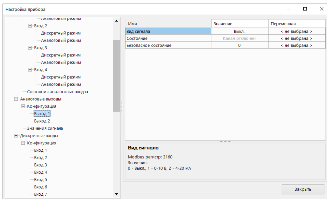
Рисунок 4.16 – Настройка универсальных аналоговых выходов
