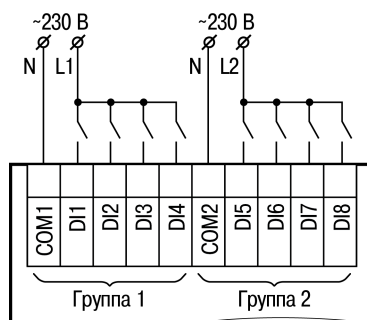
Рисунок 6.9 – Схема подключения дискретных датчиков с питанием 230 В к входам типа «ДФ»
