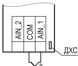
Рисунок 6.3 – Подключение ТП
