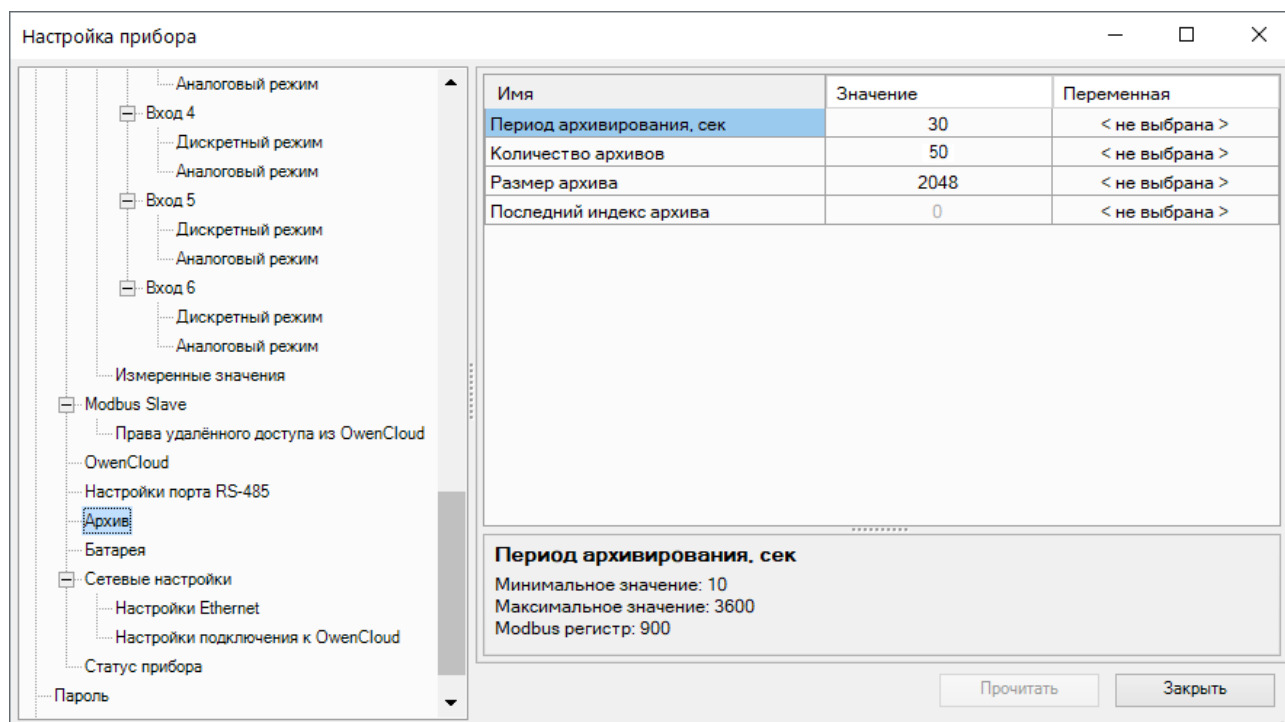
Рисунок 4.13 – Настройка параметров архива
