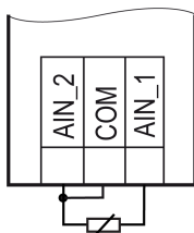
Рисунок 6.1 – Подключение ТС и других резистивных датчиков по трехпроводной схеме
