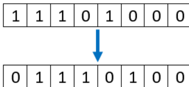
Рисунок 3.12 – Сдвиг вправо, n=1
