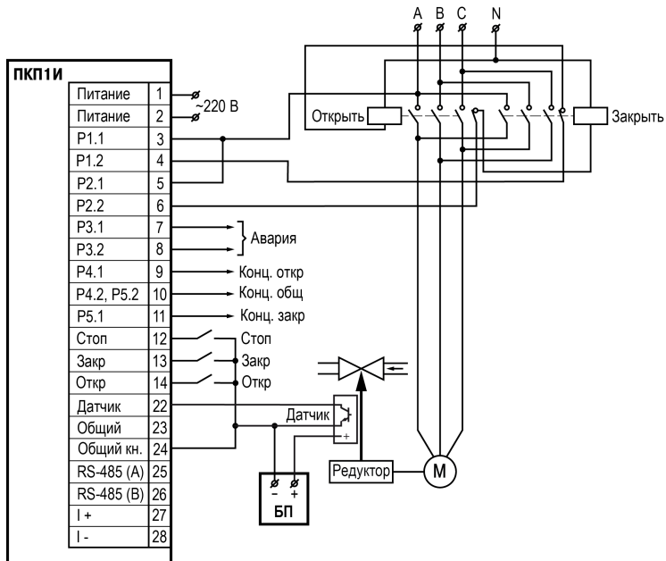
Рисунок Б.3 – Схема подключения прибора к редуктору с трехпроводным датчиком
