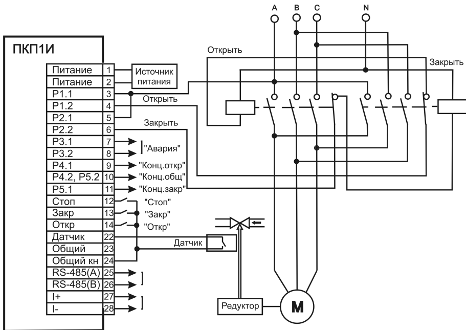
Рисунок Б.2 – Схема подключения прибора к редуктору с двухпроводным датчиком
