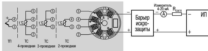
Рисунок 6.3 – Подключение прибора
