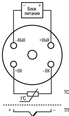
Рисунок 6.2 – Подключение прибора
