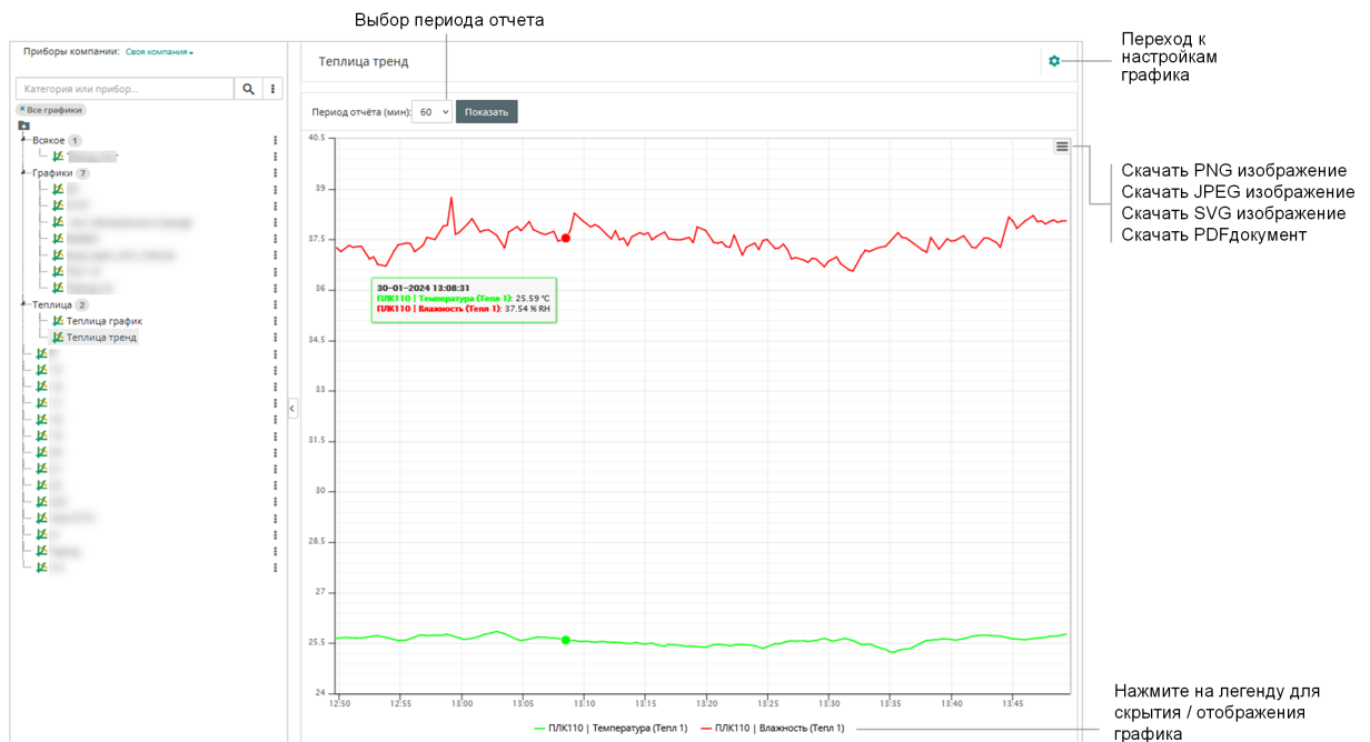
Рисунок 9.2 – Тренд
