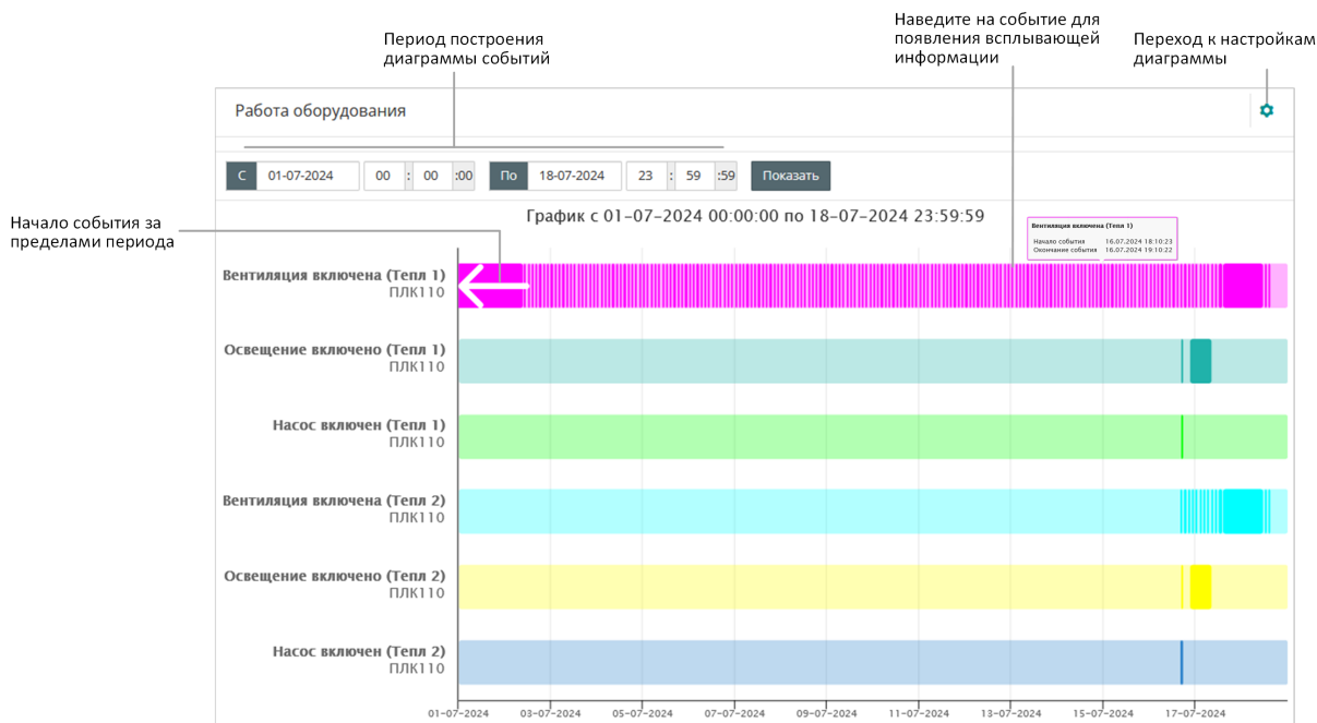
Рисунок 9.3 – Диаграмма событий
