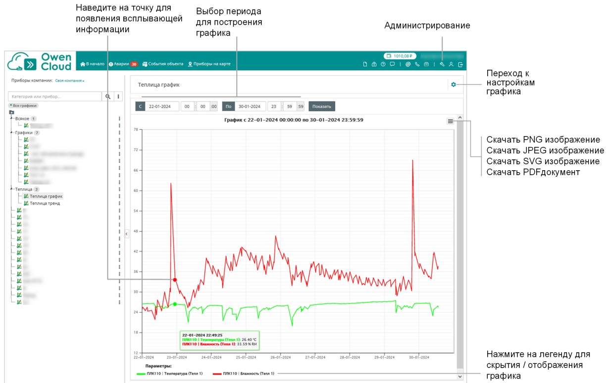
Рисунок 9.1 – Пользовательский график
