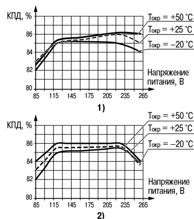
Рисунок 7 - График зависимости КПД от напряжения питания и температуры окружающей среды: (1) БП60А-12, (2) БП60А-24
